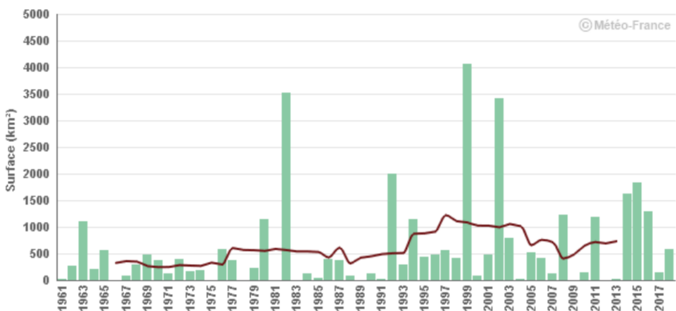
Figure 1.8. Évolution observée de la surface maximale impactée par des précipitations supérieures à 200 mm/jour sur le Languedoc-Roussillon. La courbe en rouge représente la moyenne glissante des données annuelles par périodes de 11 ans.
