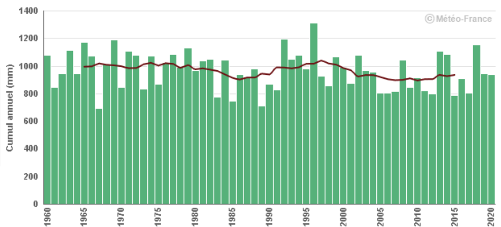
Figure 1.2. Évolution du cumul annuel des précipitations (mm) en moyenne sur la région de 1960 à 2020. La courbe en rouge représente la moyenne glissante des données annuelles par périodes de 11 ans.
