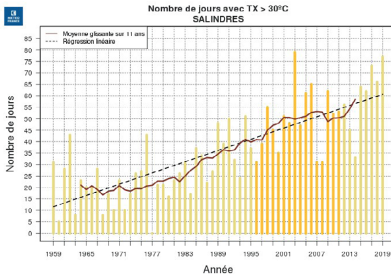
Figure 7.6. Nombre de jours très chauds (température maximale supérieure à 30 °C) à Salindres, Gard. (Source : Météo-France, dans GREC-Sud et RECO, 2020 ).
