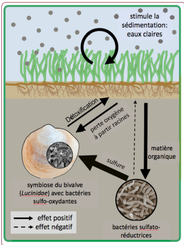
Figure 6.12. Schéma des interactions écologiques et biogéochimiques au sein d'un sédiment d'un herbier de zostères naines ( Zostera noltei ).
