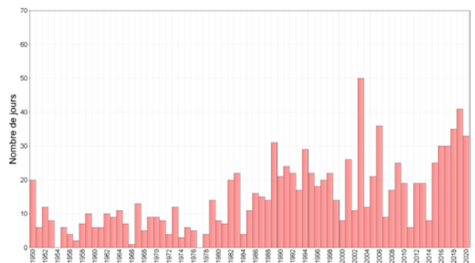
Figure 1.5. Évolution du nombre annuel de nuits tropicales à Nîmes de 1950 à 2020
