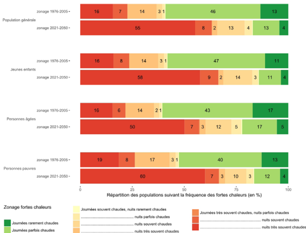
Figure 4.2. Répartition de la population et des sous-populations vulnérables en 2017 suivant la zone climatique du territoire de résidence. Sur la période 1976-2005, 16 % de la population habitait des zones avec des journées estivales et des nuits tropicales très fréquentes. Sur la période 2021-2050, cette part pourrait atteindre 55 % de la population. (Source : Insee, Fichier démographique sur les logements et les individus 2017 (Fidéli) dans INSEE , 2020)
