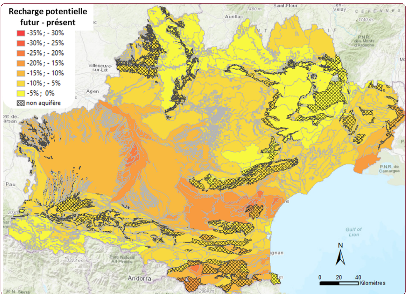
Figure 3.5. Anomalies moyennes des projections de recharge potentielle moyenne annuelle entre les valeurs futures à l’horizon 2050 (2041-2060) et présentes (1981-2010) calculées à partir de 5 projections climatiques issues de CMIP5 (Taylor et al., 2012), régionalisées de deux manières différentes (Pagé et al., 2009 ; Dayon, 2015) - Fond de carte : World topographic map – ©ArcGIS.. (Source : Caballero, 2021, pour le CROCC)
