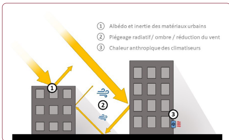
Figure 5.5. Influence du bâti sur le confort extérieur, principaux mécanismes. (Source : réalisation de M. Bonhomme)
