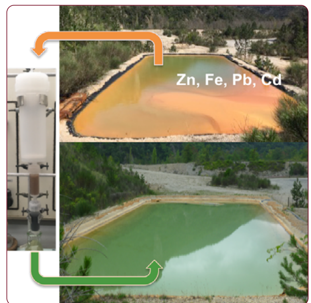
Figure 4.5. Dépollution des eaux minières (Malines/Gard) par le filtre végétal ChimEco/Bioinspir. (Source : C. Grison)
