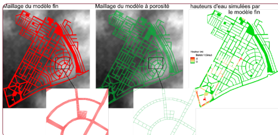
Figure 5.8. Comparaison d'un modèle classique et à grandes mailles en milieu urbain pour une pluie de 4h. Les durées de calcul sont de 4h environ pour le modèle fin et 2min pour le modèle « à porosité ». Bien que moins précis, les résultats du modèle à porosité sont du même ordre de grandeur (Source : modèles développés par des chercheurs des laboratoires HSM et IMAG, membres de l'équipe Inria Lemon)
