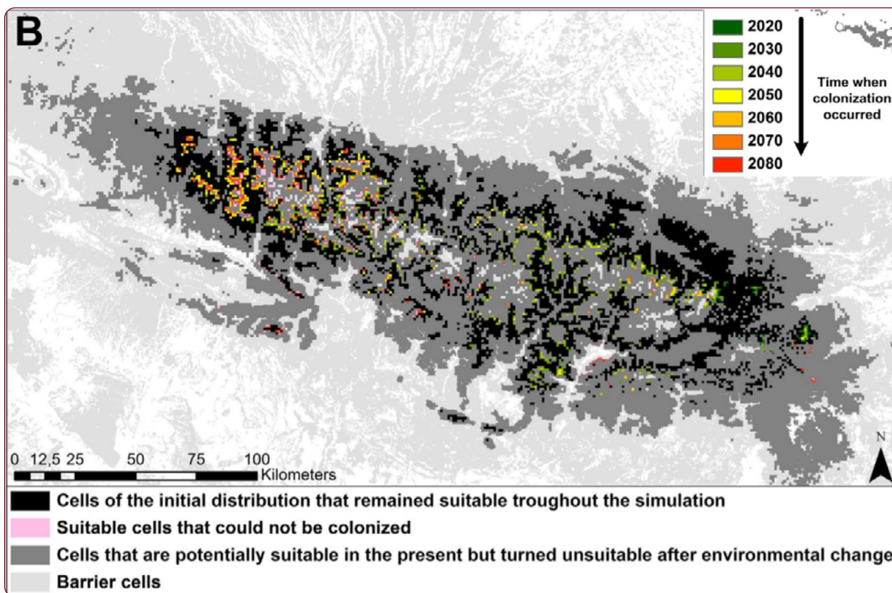
Figure 7.11. Évolution estimée de la répartition potentielle de Calotriton asper dans la chaîne pyrénéenne en 2080 par rapport à la répartition actuelle, en utilisant la moyenne des trois modèles de circulation mondiale (GCM : CCCMA, HADCM3 et CSIRO) et le scénario d'émissions SRES A2. (Source : d'après de Pous et al., 2015 dans OPCC, 2018)
