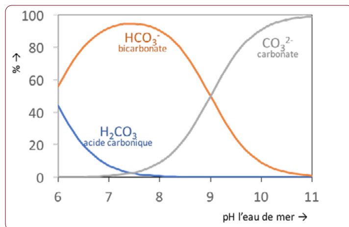
Figure 6.7. Equilibre des carbonates inorganiques dissous – proportion des trois différentes formes en fonction du pH dans l'eau de mer à 20 °C. (Source : De Wit, 2021, pour le CROCC_2021)
