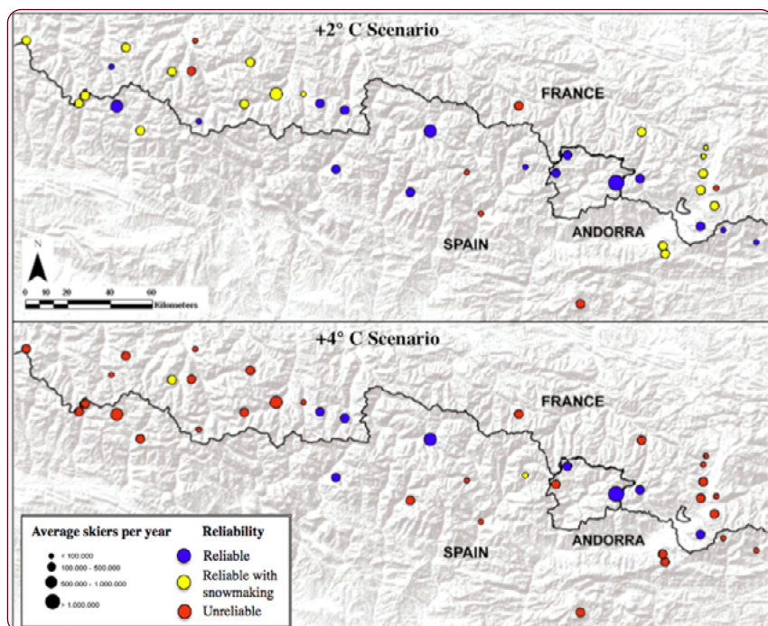
Figure 7.7. Évolution de la capacité à fonctionner des stations de ski des Pyrénées avec et sans production de neige artificielle, pour deux horizons temporels et scénarios futurs différents (+2 °C, pour 2051-2070, et +4 °C pour 2071-2100). (Source : Pons et al., 2015 dans OPCC, 2018).
