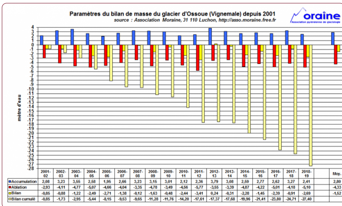
Figure 7.10. Bilan de masse du glacier d'Ossoue depuis 2001. (Source : Association Moraine).
