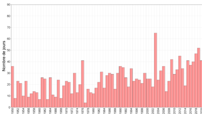
Figure 1.4. Évolution du nombre annuel de jours de forte chaleur à Toulouse de 1950 à 2020
